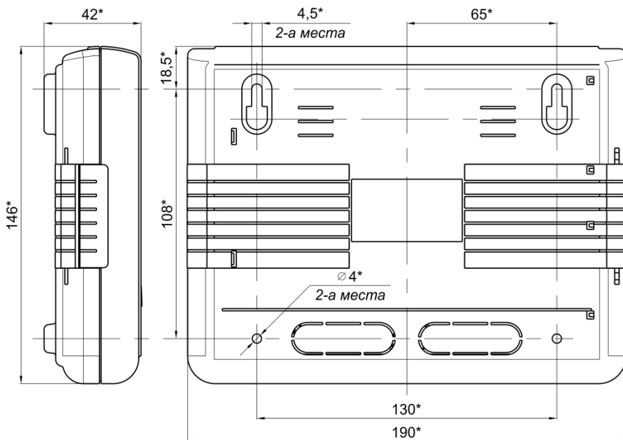
Рис 2. Габаритные и установочные размеры «BC-УРС ВЕКТОР»
